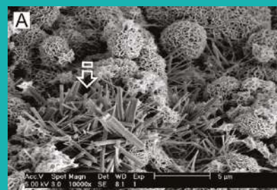
Cristalli precipitati di fosfato di calcio sparsi sulla superficie di silicato tricalcico idratato 1
